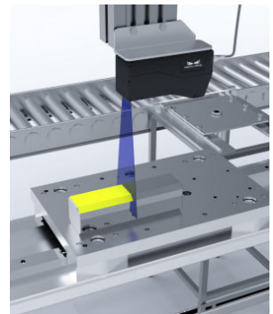
사각 실리콘 막대 평탄도 검사
