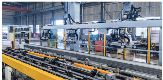
산형강 처리
